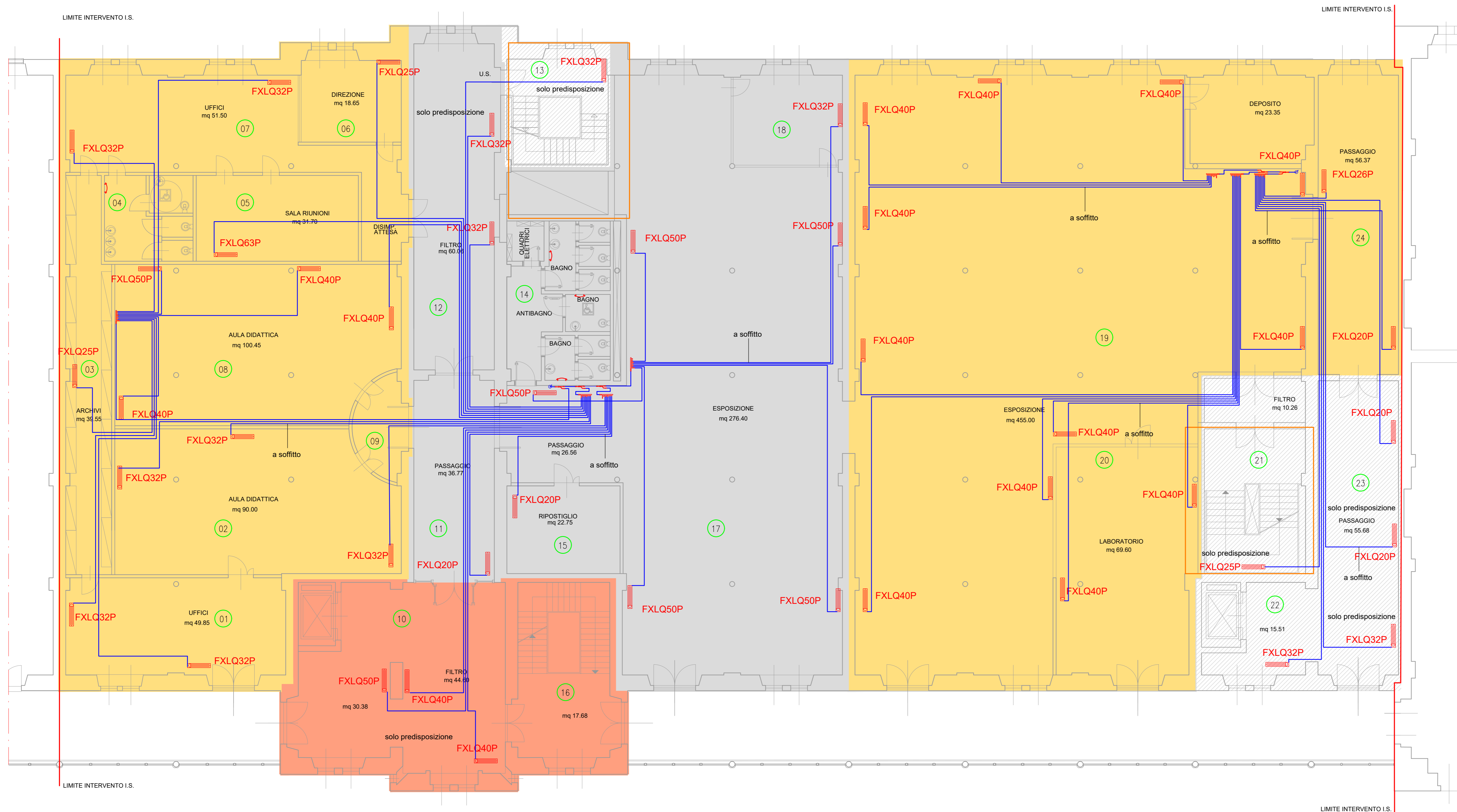
PIANTA PIANO PRIMO SCALA 1:100
