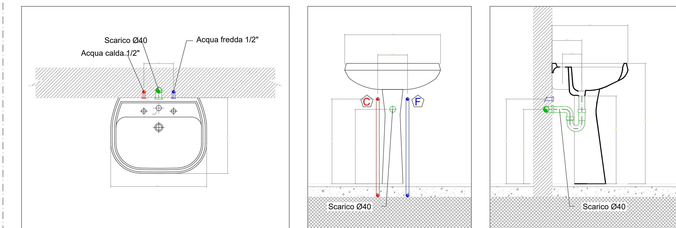
Particolare attacchi LAVANDINO scala 1:10
