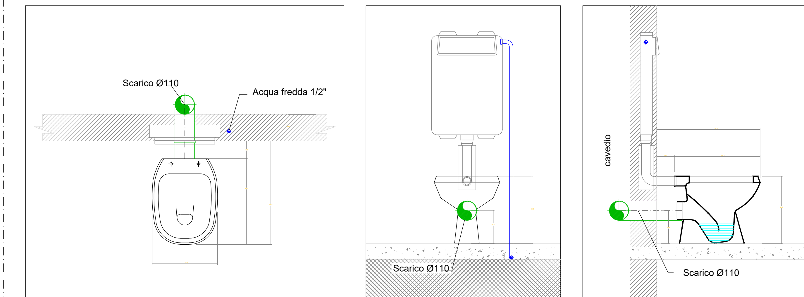
SEZ. A-A' scala 1:25
