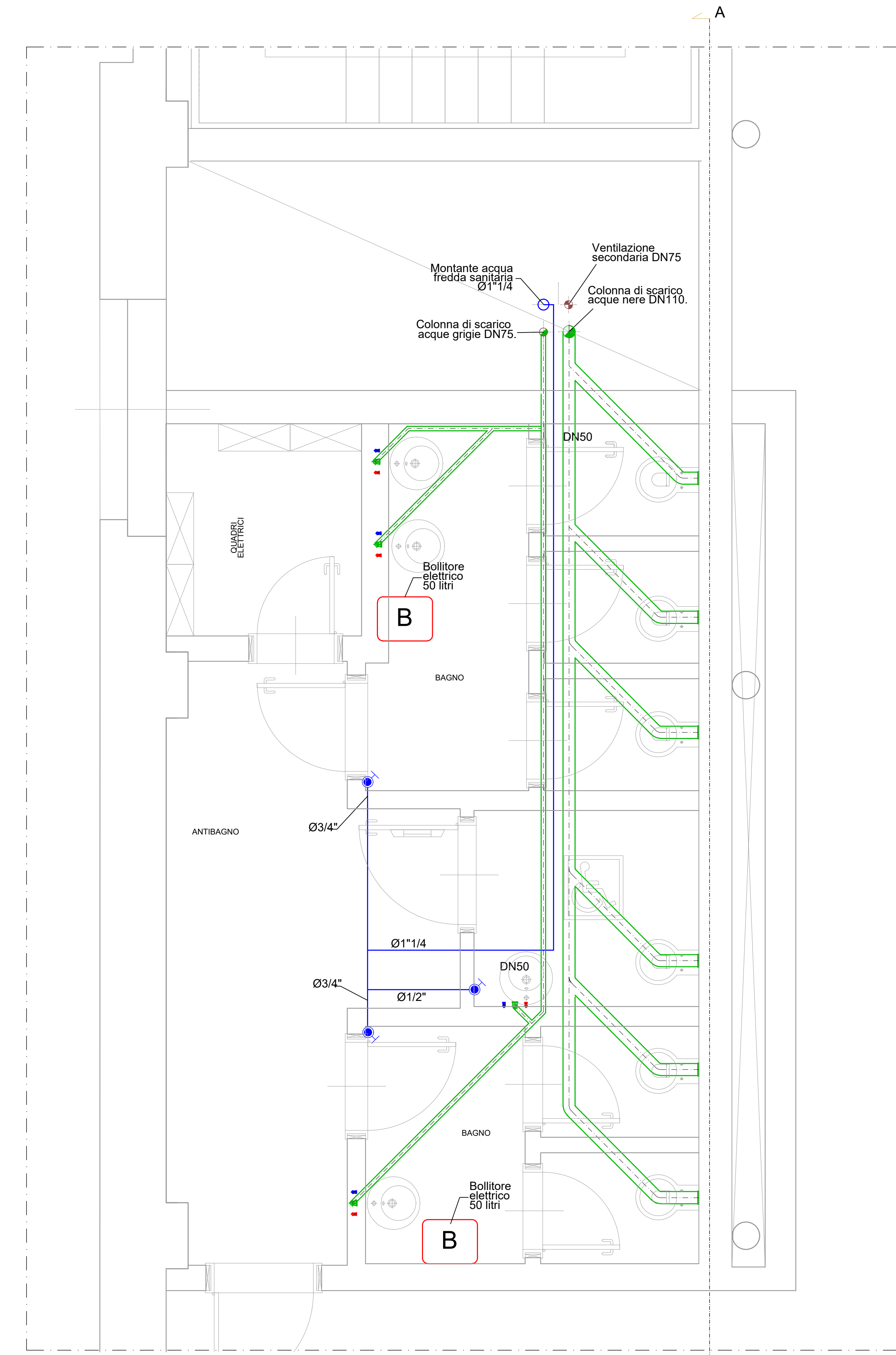
PIANTA PIANO TERZO scala 1:25
