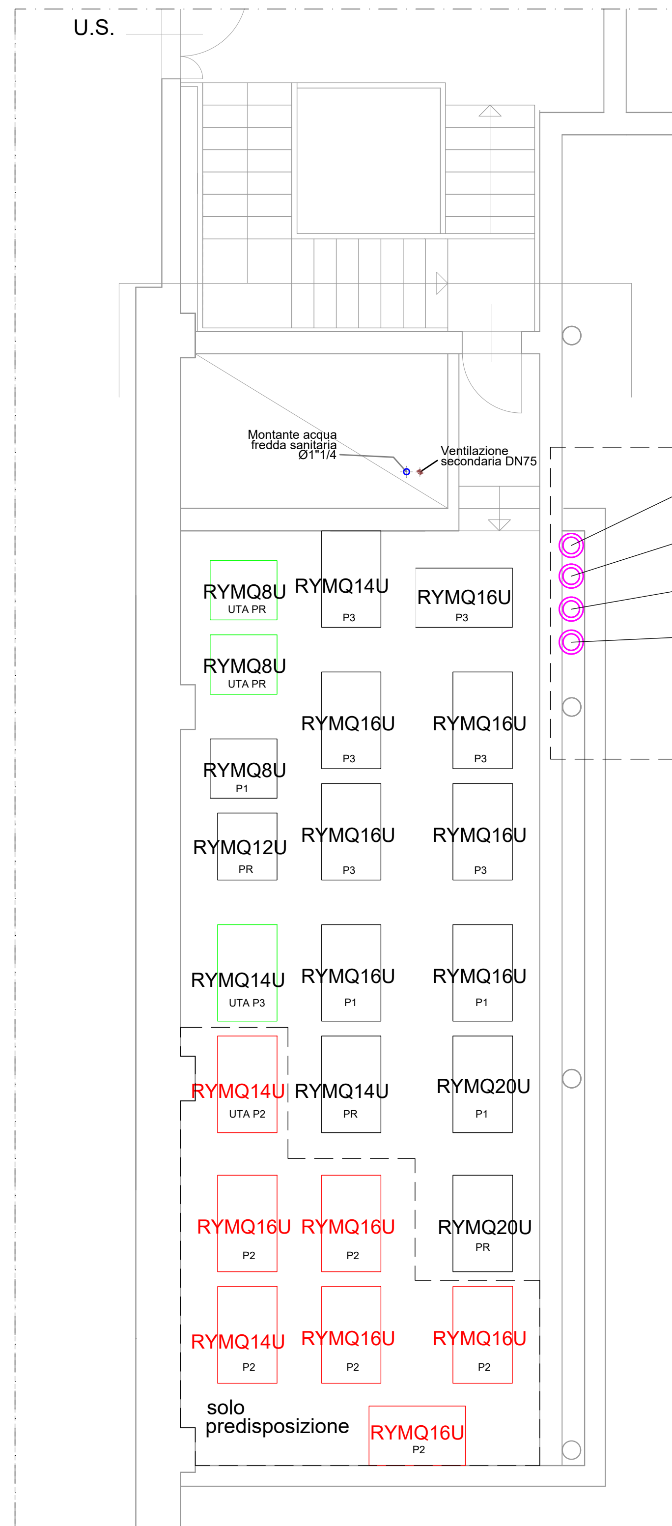
SOPPALCO IMPIANTI posizionamento unità esterne scala 1:50
